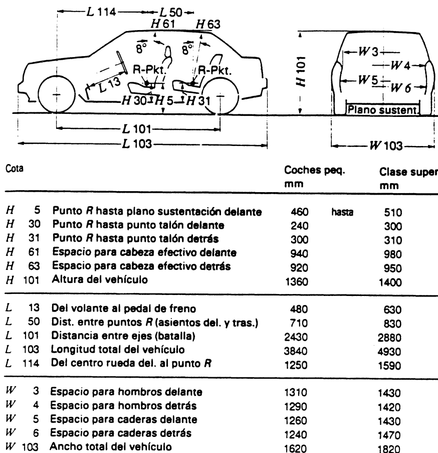
Figura 8.7. Medidas interiores y exteriores típicas
